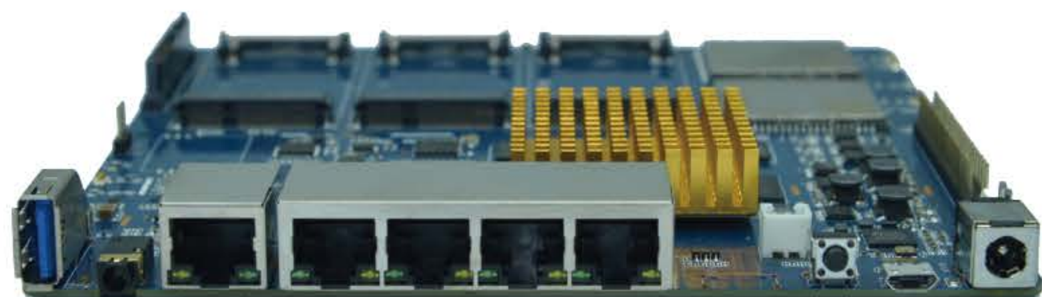
智能融合通信设备MNF-410 4卡聚合、工业级WIFI，可内置电池、视频编码板。
